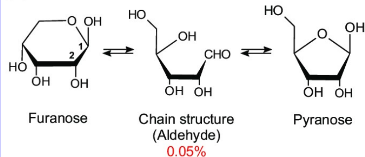
(b) D-ribose
