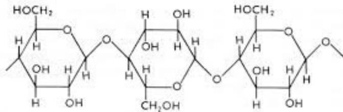
Celulóza (polysacharid)
