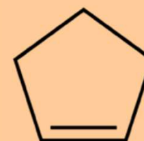
cyklopent en
