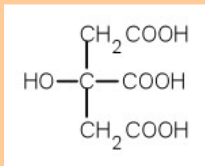
kyselina citronová
