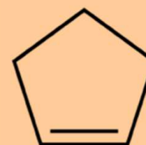
cyklopent en
