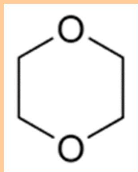
dioxan
