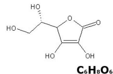
Vitamín C
