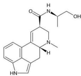
Ergometrine
