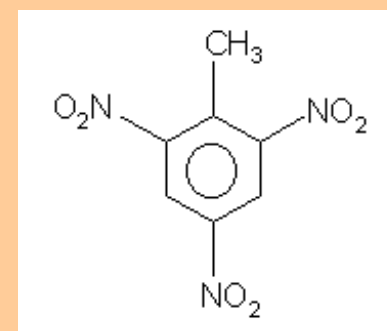
Složení Semtexu
