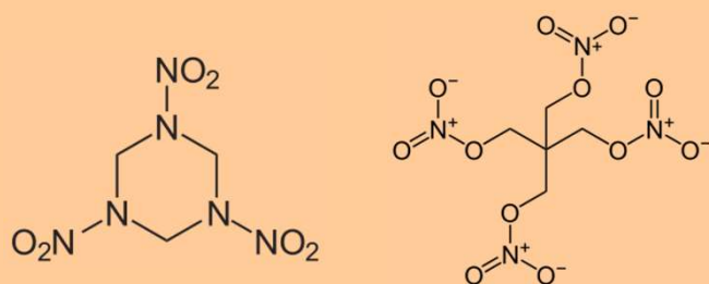
pentrit
