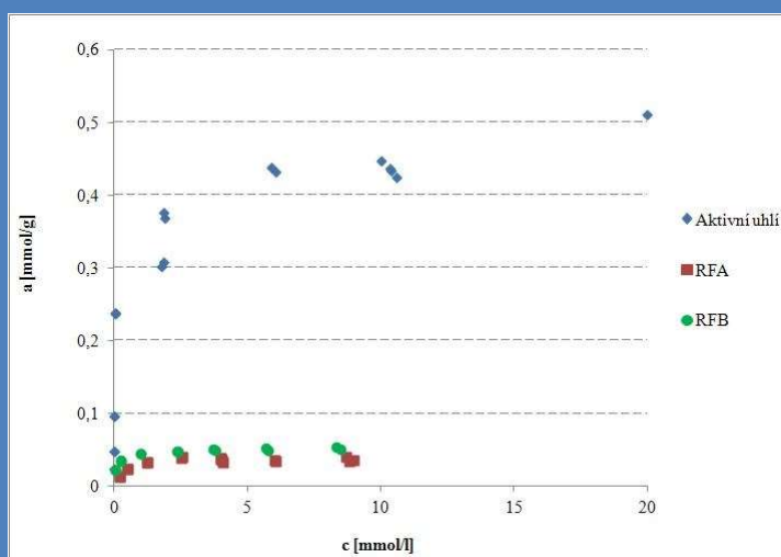
Sorpce olova ( Pb^{2+} ) na různé uhlíkové sorbenty jako funkce koncentrace
