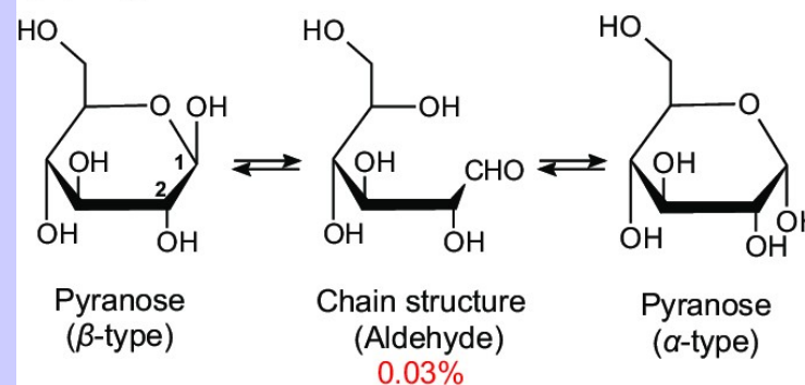
(b) D-ribose
