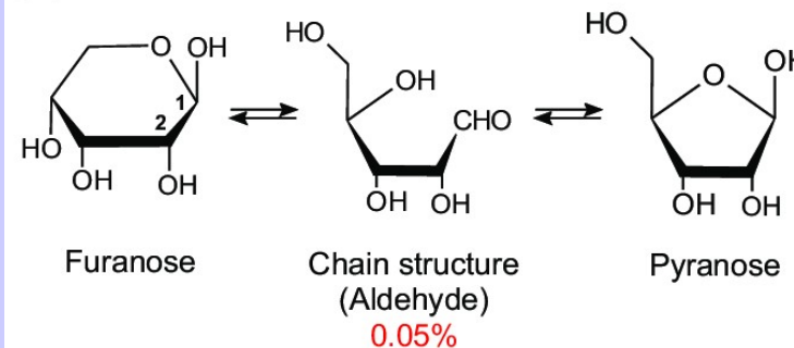
(b) D-ribose
